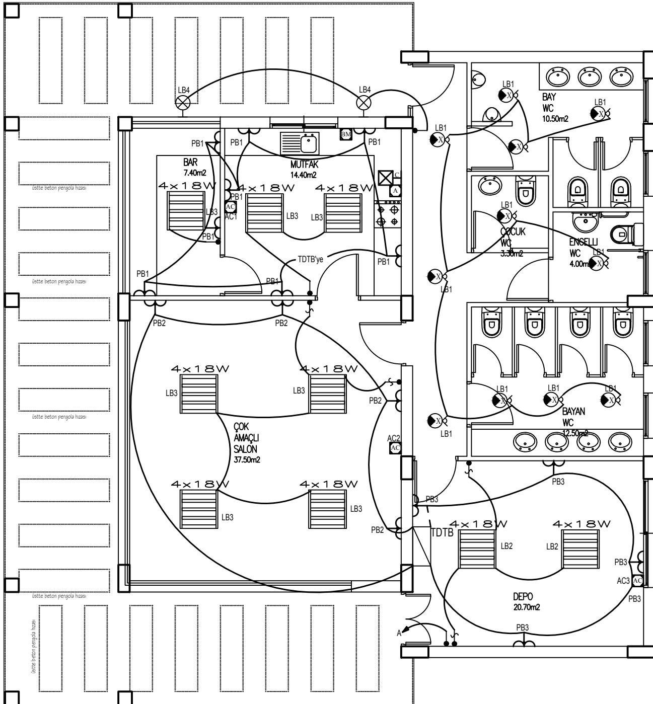
BÜFE ZEMİN KAT ÖLÇEK 1/50
