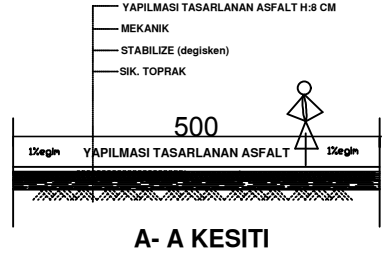
A- A KESİTİ
